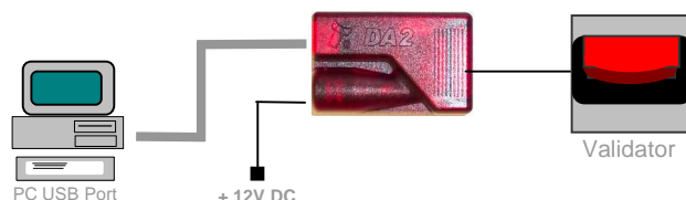
Рисунок 21 - Подключение DA2 к NV9 и PC для перепрограммирования
