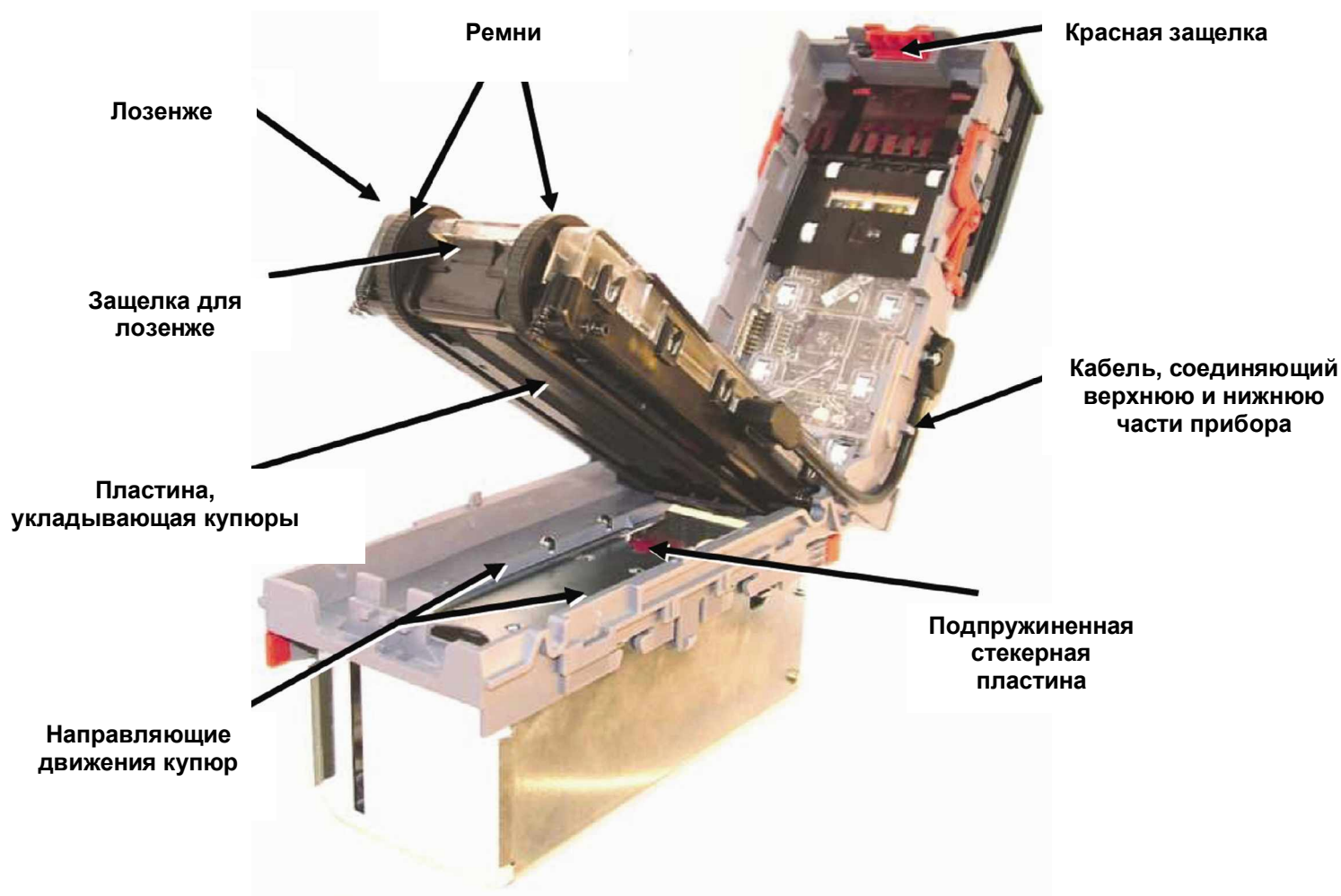
Рисунок 13 – Доступ к внутренним частям NV9
