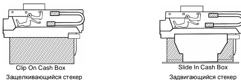
Рисунок 11 – Зашелкивающийся и задвигающийся стекер.
