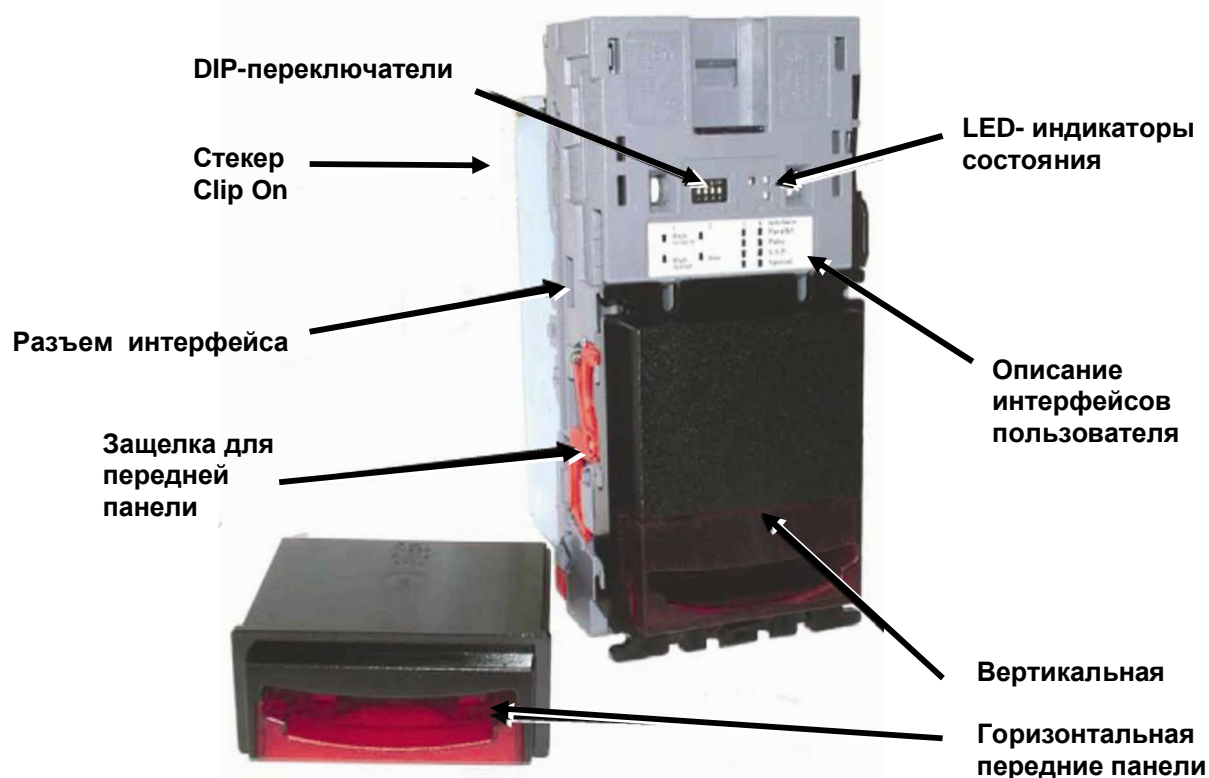
Рисунок 1 – Банкнотоприемник NV9 с вертикальной и горизонтальной передними панелями
